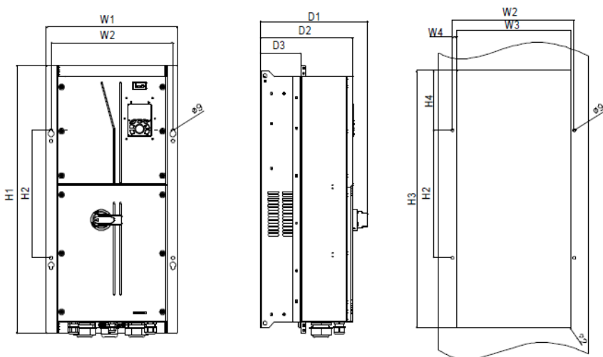
Рис С.4 Схема фланцевого монтажа ПЧ моделей 045G/55P–055G/075P
